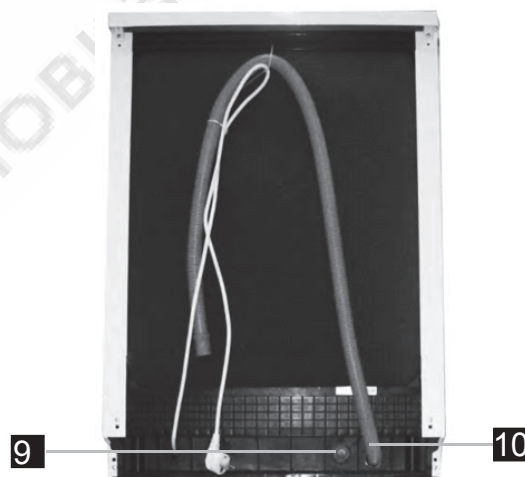
Вид сзади
